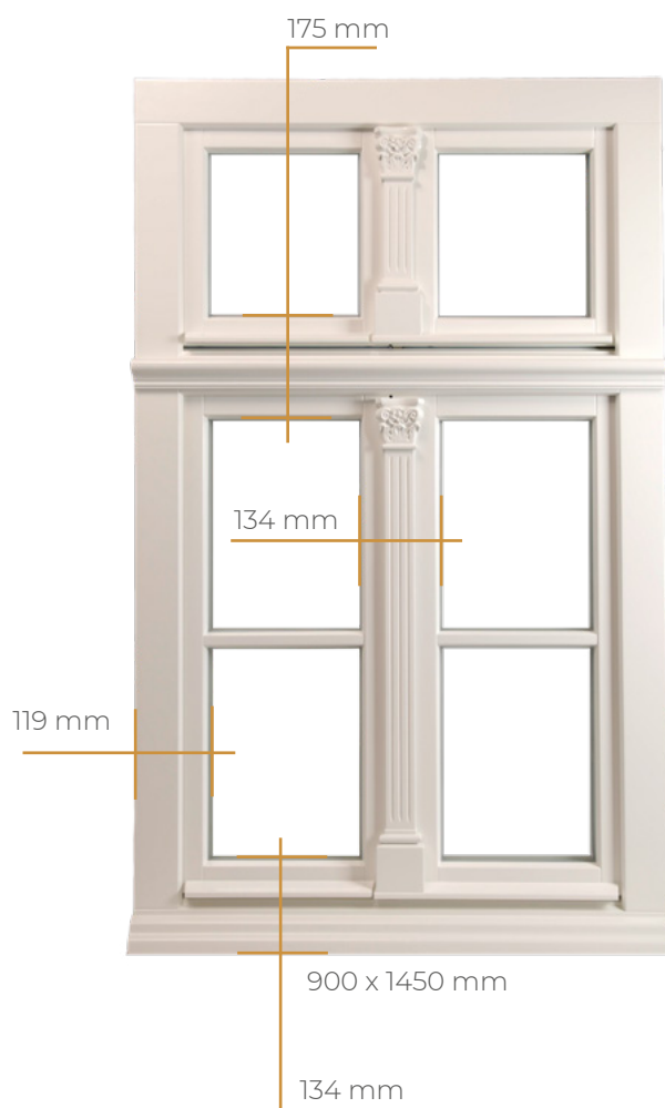
STANDARDPROFIL
